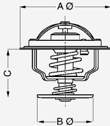
Typ A B C 4006 54 35 33 mit Entlüftungsventil 4026 54 28 30 mit Positionskerbe 4029 54 29 32 mit Entlüftungsventil 4033 56 34 33 ohne Entlüftungsventil oder -Kerbe 4154 54 29 32 mit Entlüftungsventil 4253 54 35 31 Ventilteller gummi- beschichtet 4256 54 35 31 ohne Entlüftungsventil oder -Kerbe 4272 54 35 31 mit Entlüftungsventil
