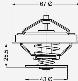
Typ 4030 mit Entlüftungskerbe 4059 4064 mit Entlüftungsventil kühlenseitig 4078 mit Entlüftungsventil motorseitig 4083 mit Entlüftungskerbe 4112 mit Entlüftungsventil 4122 mit Entlüftungsventil 4158 mit Entlüftungsventil
