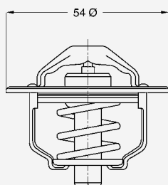
Typ 3116 mit Entlüftungsventil
