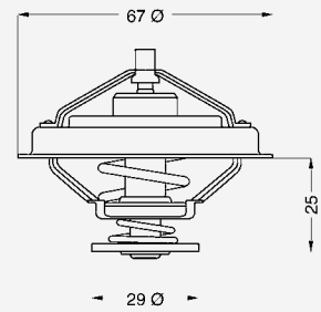
Typ 4166 mit Entlüftungsventil
