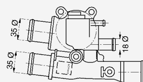
Typ 3163 mit M 12 x 1,5 Typ 3481 mit M 12 x 1,5 / M 16 x 1,5
