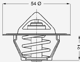
Typ 3023 mit Entlüftungskerbe
