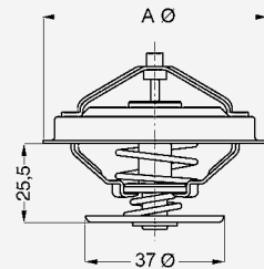
Typ A B 4049 67 37 ohne Entlüftungsventil oder -kerbe 4088 67 37 ohne Entlüftungsventil oder -kerbe 4132 75 43 mit Entlüftungskerbe 4116 67 37 Ventilteller gummi- beschichtet 4117 67 37 mit Entlüftungskerbe
