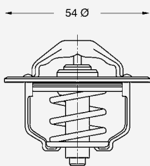
Typ 3103 mit Entlüftungsventil
