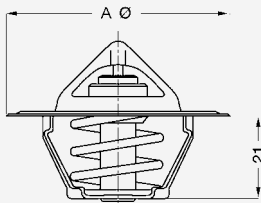
Typ A 3000 54 mit Entlüftungskerbe 3021 48 3044 44 3136 53,5 3141 54 ohne Entlüftungskerbe 3167 54 gummibeschichtete Ventilplatte
