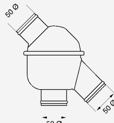
Typ 4663 4684 mit Entlüftungsventil
