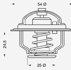
Typ 4003 ohne Entlüftungsventil oder -kerbe 4008 mit Entlüftungsventil 4015 mit Entlüftungsventil
